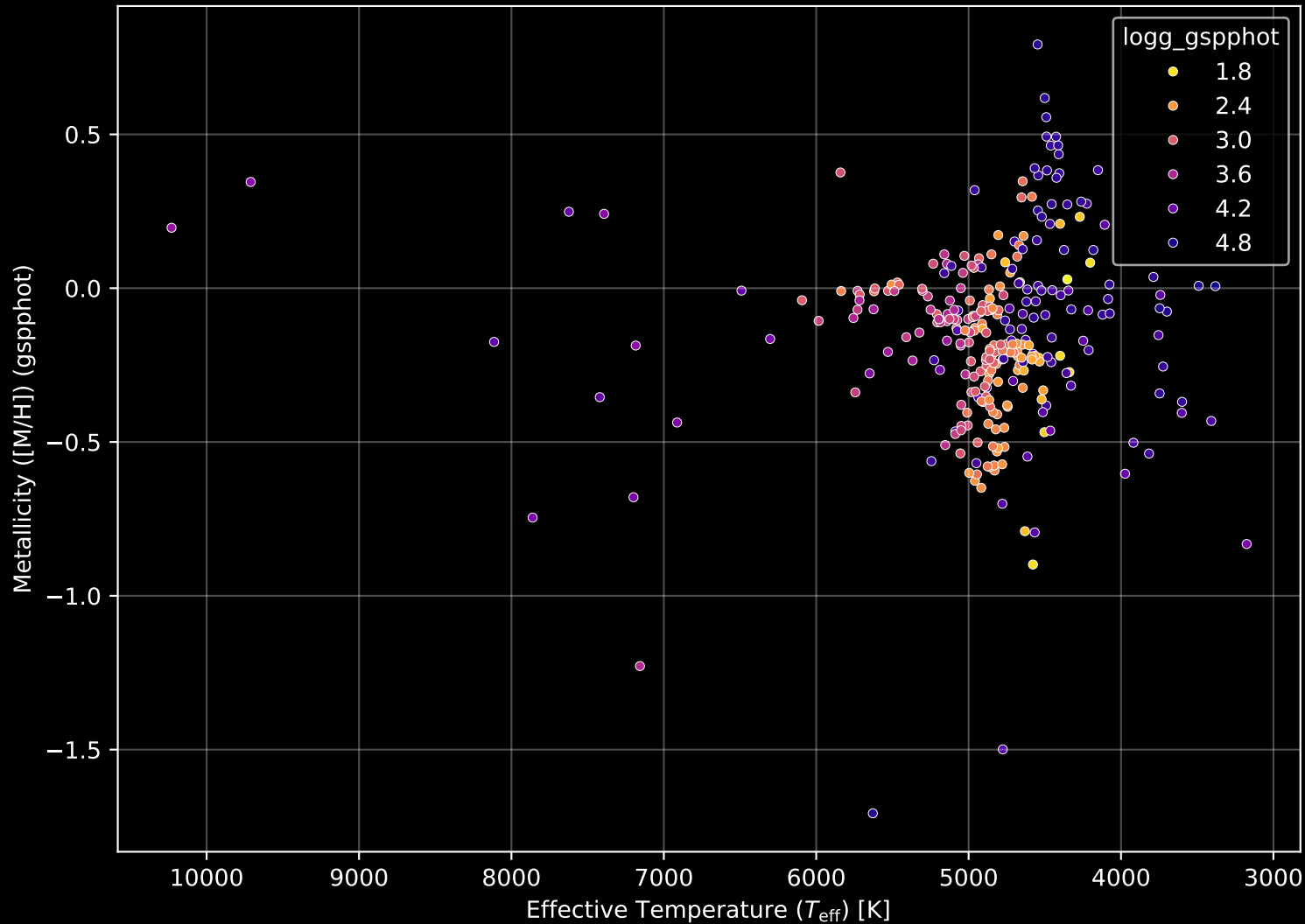
APOGEE DR17 Field: [201+30_btx] Stellar Population Parameters (n= 297)
